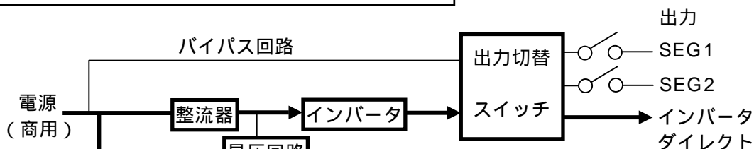
指定セグメントコンセント停止時の電力供給経路
