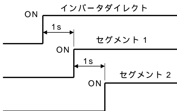
セグメントディレーON タイミング(デフォルト)
