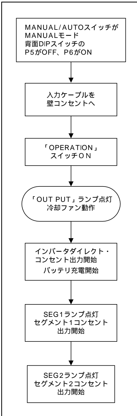
セグメントディレー制御運転時の電力供給経路
