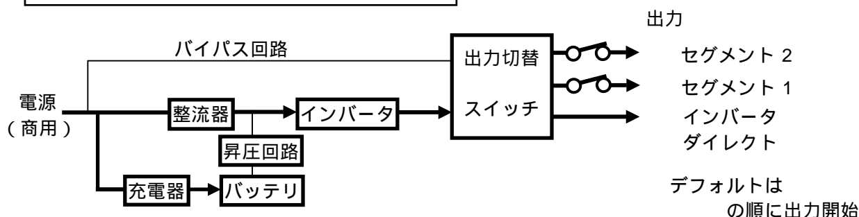
セグメントディレー制御運転時の電力供給経路
