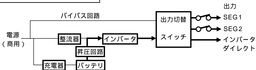
商用電源異常時の電力供給経路
