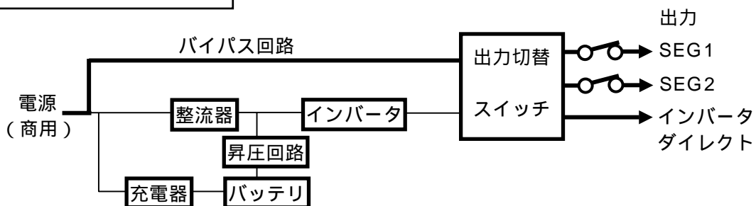
重故障時の電力供給経路
