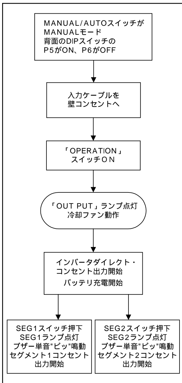
セグメント独立制御運転時の電力供給経路
