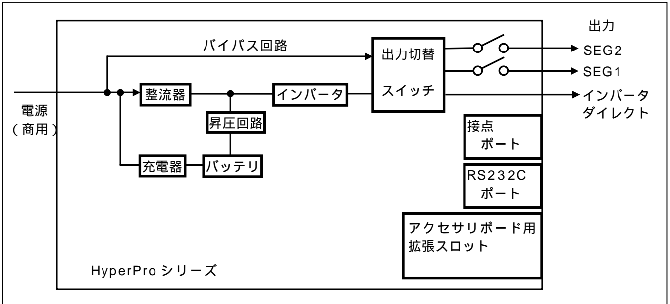
HyperPro シリーズ概略構成図
