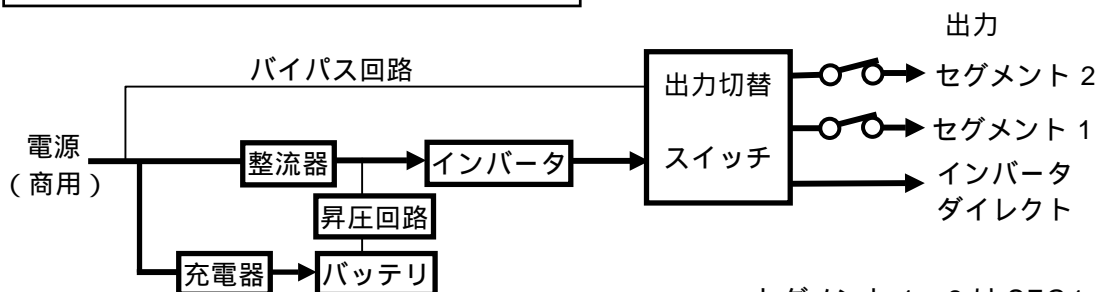
セグメント独立制御運転時の電力供給経路
