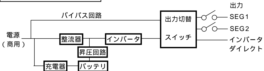
過負荷停止時の電力供給経路
