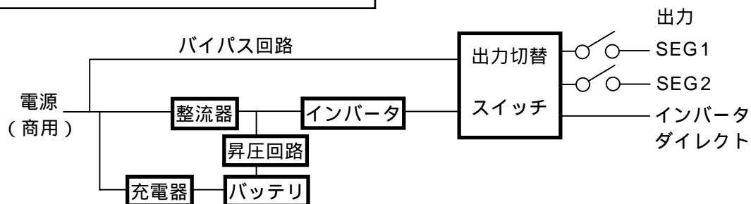
全出力コンセント停止時の電力供給経路
